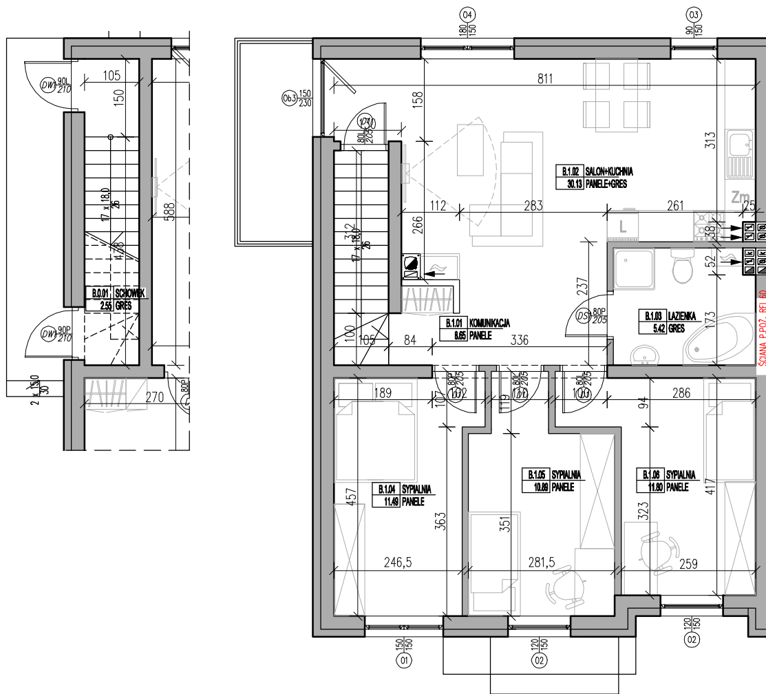
RZUT PARTERU LOKAL B
