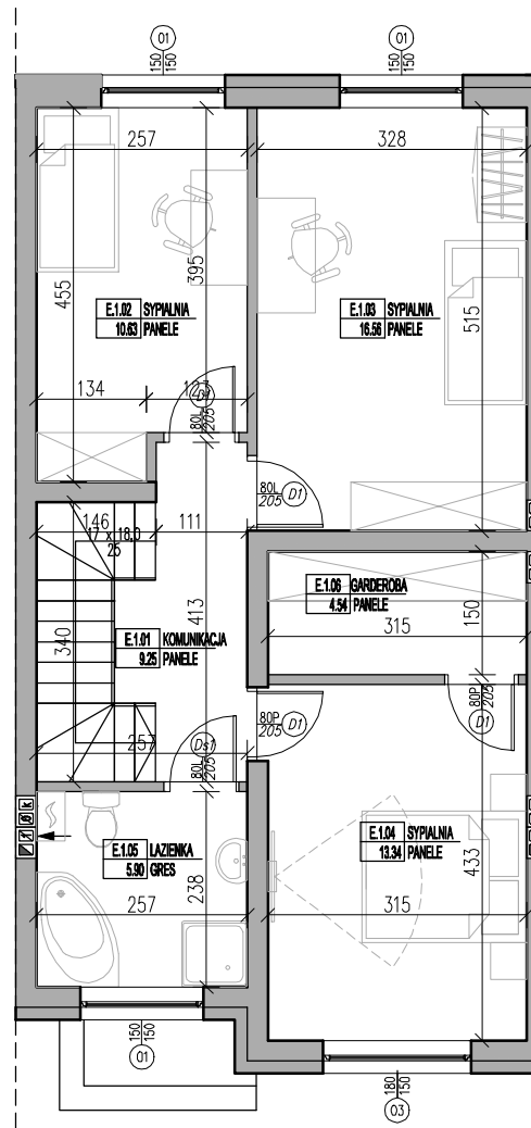
RZUT PIĘTRA LOKAL E
