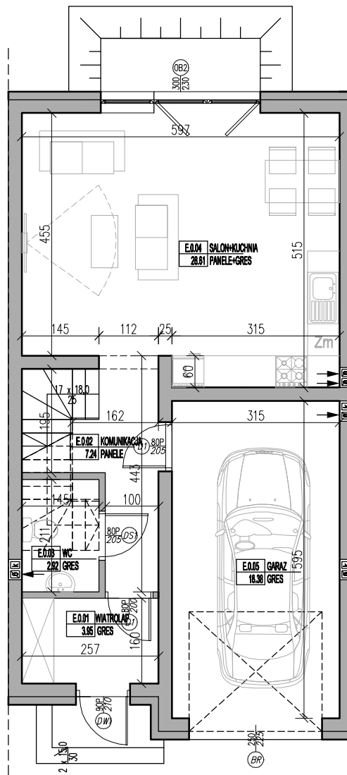
RZUT PARTERU LOKAL E
