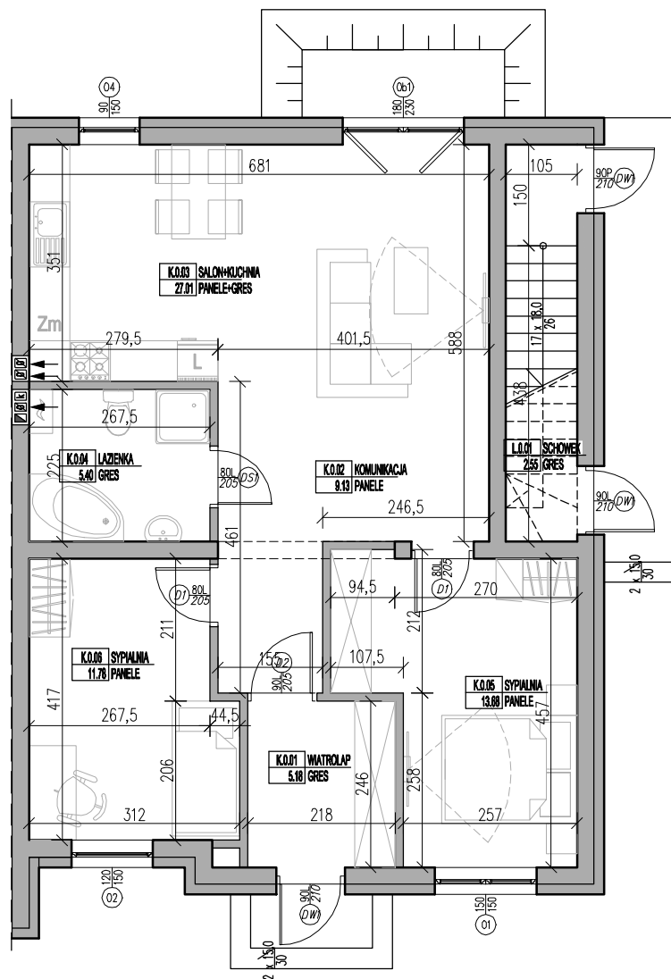
RZUT PARTERU LOKAL K
